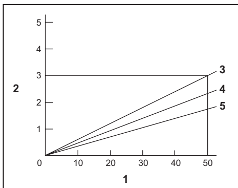
1. Frecuencia de clavado (veces/min) 2. Salida de aire del compresor por minuto (CFM: pies cúbicos por minuto (ft 3 /min)) 3. 0,83 MPa (120 PSIG) 4. 0,66 MPa (95 PSIG) 5. 0,49 MPa (70 PSIG)
