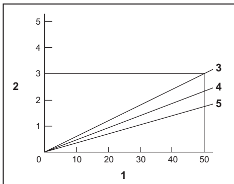
1. Fréquence de clouage (fois/min) 2. Sortie d'air du compresseur par minute (CFM (ft³/min)) 3. 0,83 MPa (120 PSIG) 4. 0,66 MPa (95 PSIG) 5. 0,49 MPa (70 PSIG)
