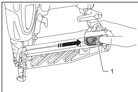
► 1. Levier-poussoir
